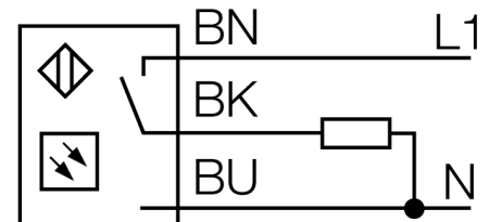
Anschlussbild
